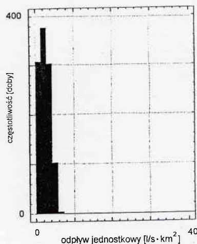
RYСУNEK 4. Częstość średnich dobowych odpływów jednostkowych zlewni Strugi Dormowskiej do przekroju Gorzyń w latach hydrologicznych 1987/88–1989/90
