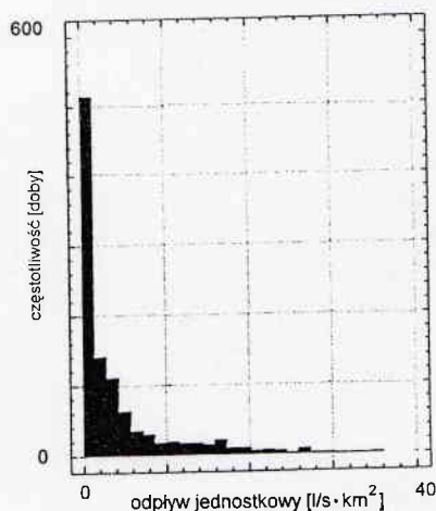
RYСУNEK 3. Częstość średnich dobowych odpływów jednostkowych zlewni Maskawy do przekroju Dzierznica w latach hydrologicznych 1987/88–1989/90
