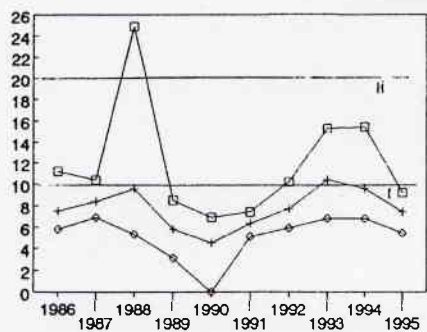
RYSUNEK 5. Maksymalne (□), średnie (+) i minimalne (◇) roczne wartości oznaczeń tlenu rozpuszczonego, BZT 5 i utlenialności w wodach rz. Strugi Dormowskiej w Gorzynie i rz. Maskawy w Dzierżnicy
