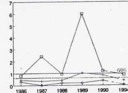
RYSUNEK 7. Maksymalne (□), średnie (+) i minimalne (○) roczne wartości oznaczeń azotu amonowego, azotu azotanowego i fosforanów w wodach rz. Strugi Dormowskiej w Gorzynie i rz. Maskawy w Dzierżnicy
