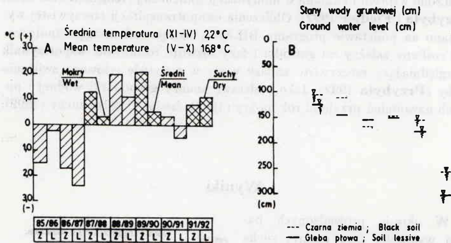
Ryc. 2. Odchylenia półrocznych temperatur (A) od średnich z wielolecia oraz stany wody gruntowej (B) w czarnych ziemiach i glebach płowych w latach 1987-1992 Fig. 2. Deviation of mean half-year temperatures (A) from multiyear mean and ground water level in years 1987-1992
