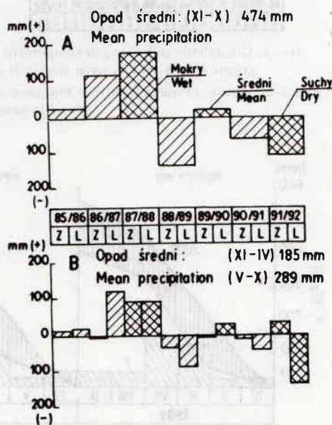
Ryc. 1. Odchylenia rocznych (A) i półrocznych (B) sum opadów od średnich z wielolecia 1986-1992
