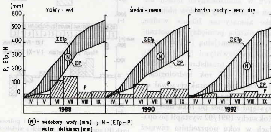
Ryc. 3. Miesięczne sumy opadów (P) oraz krzywe sumowania opadów (ΣP), ewapotranspiracji potencjalnej (ΣETp) i wielkość niedoborów wody (N) Fig. 3. Monthly sums of precipitation (P) and cumulative curves of precipitations (ΣP), potential evapotranspiration (ΣETp) and water deficiency (N)
