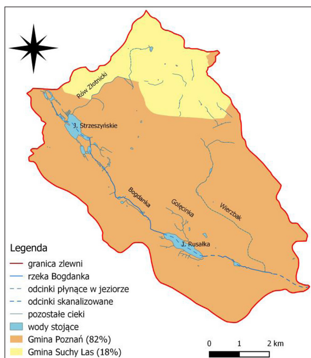
Rys. 1. Zlewnia cieków Bogdanki (na podstawie rastrowej mapy podziału hydrograficznego Polski i państwowego rejestru granic)
