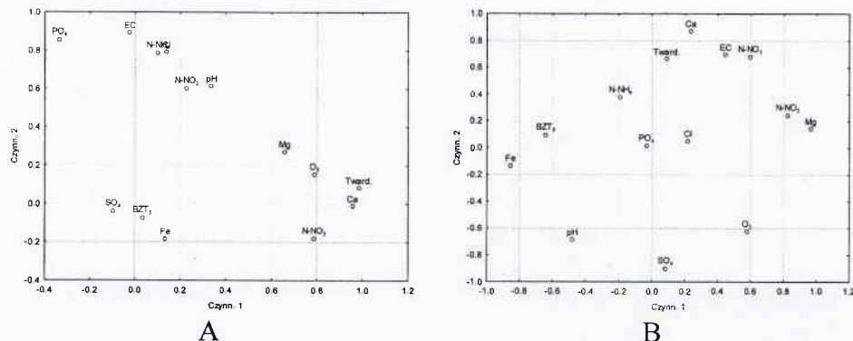
Rys. 4. Wykres rozrzutu ładunków czynnikowych względem dwóch pierwszych czynników dla wód rzek Orli i Radęcy (A) oraz zbiorników Jutrosin i Pakosław (B) Fig. 4. Scatter plot of factor loadings with respect to the first two factors for Orla and Radeca Rivers (A) and Jutrosin and Pakoslaw Reservoirs (B)
