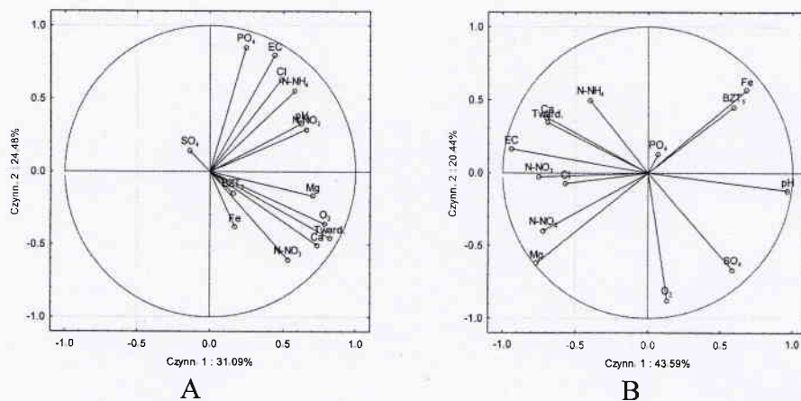
Rys. 5. Wyniki analizy składowych głównych dla wód rzek Orli i Radęcy (A) oraz zbiorników Pakosław i Jutrosin (B) Fig. 5. The results of principal components analysis for Orla and Radeca (A) Rivers due to Pakoslaw and Jutrosin Reservoirs (B)
