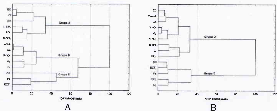
Rys. 3. Podział wskaźników jakości wody na grupy o podobnej zmienności w wodach rzek Orli i Radęcy (A) oraz zbiornikach Jutrosin i Pakosław (B) Fig. 3. Water quality factors division with similar groups for Orla and Radeca Rivers (A) due to Jutrosin and Pakoslaw Reservoirs (B)
