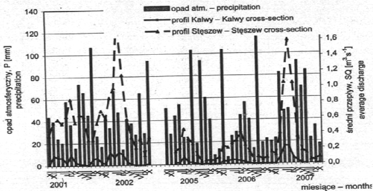
Rys. 3. Średnie miesięczne przepływy rzeki Samica Stęszewska w profilach Kalwy i Stęszew na tle opadów atmosferycznych w badanych latach hydrologicznych Fig. 3. Average monthly discharge of Samica Stęszewska River in Kalwy and Stęszew cross-section in aspect of hydrological annual precipitation
