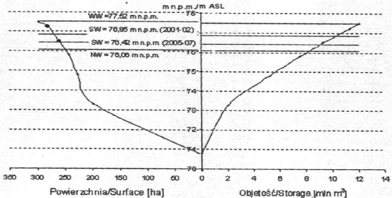
Rys. 5. Krzywe powierzchni i pojemności Jeziora Niepruszewskiego
