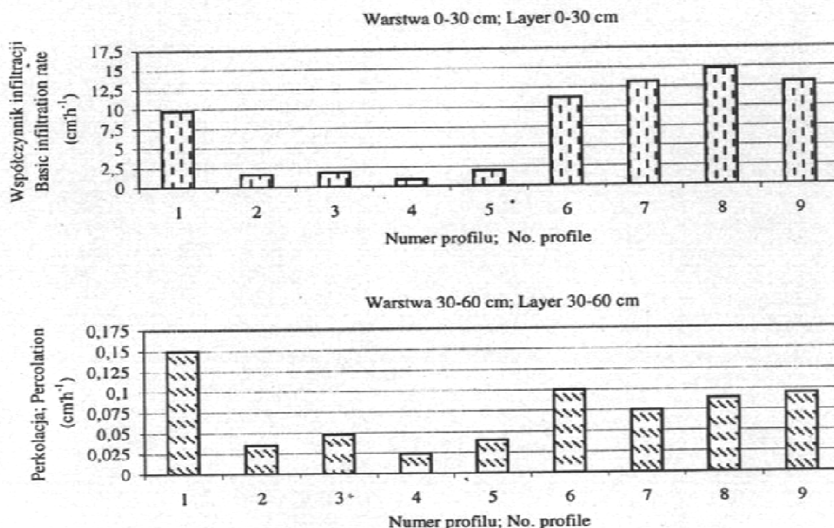
Rys. 3. Wartość współczynnika infiltracji w warstwie 0–30 cm i perkolacji w warstwie 30–60 cm w badanych profilach gruntów pogórnicych
