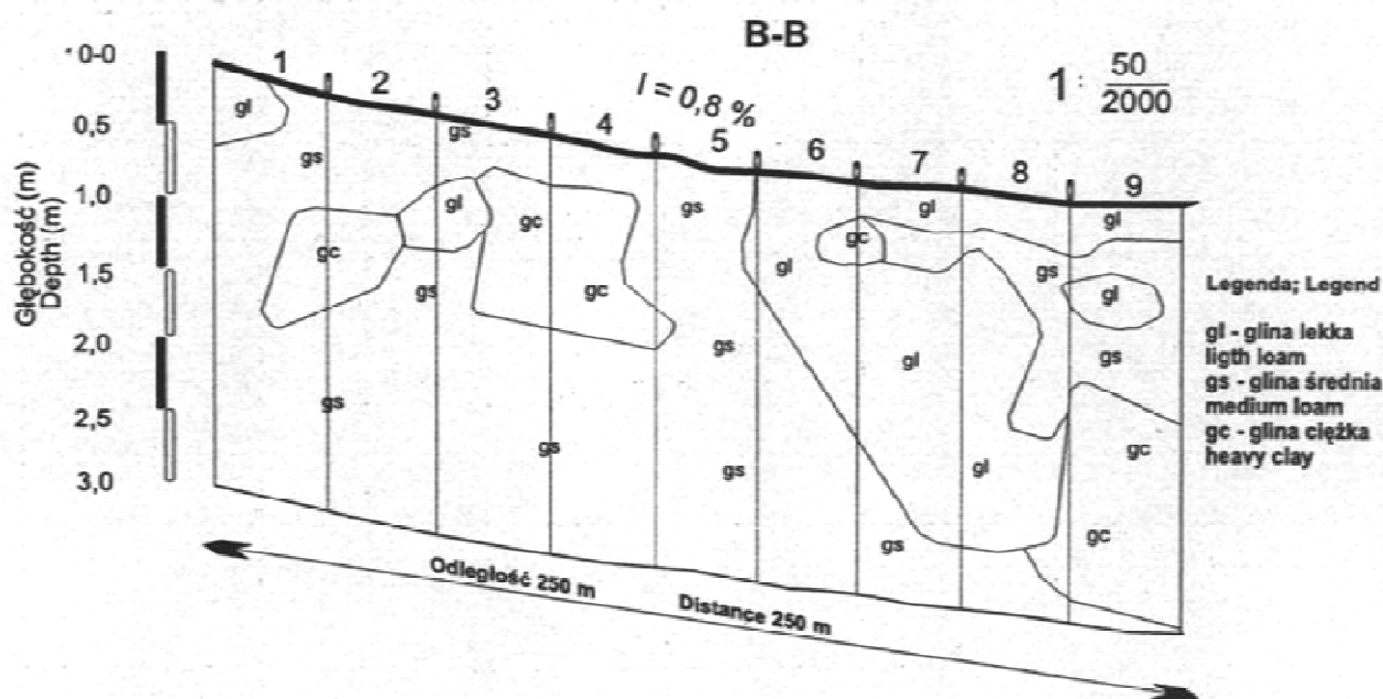
Rys. 1. Podłużny przekrój pedologiczny badanych powierzchni doświadczalnych transektu B-B
