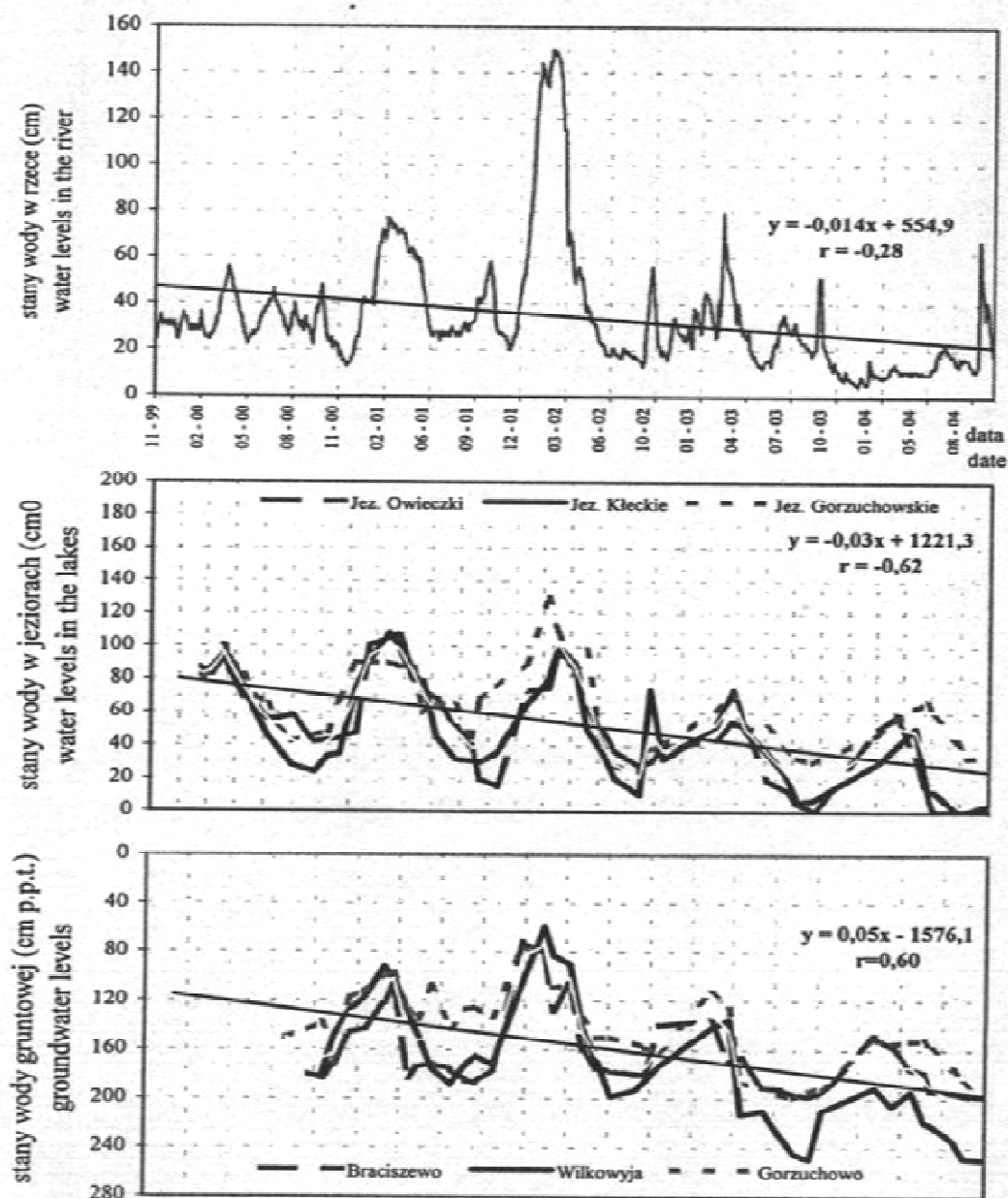
Rys. 2. Przebieg stanów wody w cieku, w jeziorach i studzienkach kontrolno-pomiarowych
