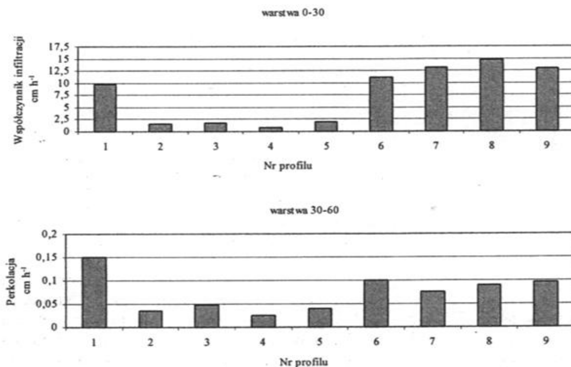
Rys. 4. Współczynniki infiltracji ustalonej w warstwie 0÷30 cm i współczynniki perkolacji w warstwie 30÷60 cm w badanych profilach gruntów pogórnich Fig. 4. Coefficients of vertical percolation in layer 0÷30 cm and coefficients of vertical percolation in layer 30÷60 cm in experimental post-mining grounds profiles
