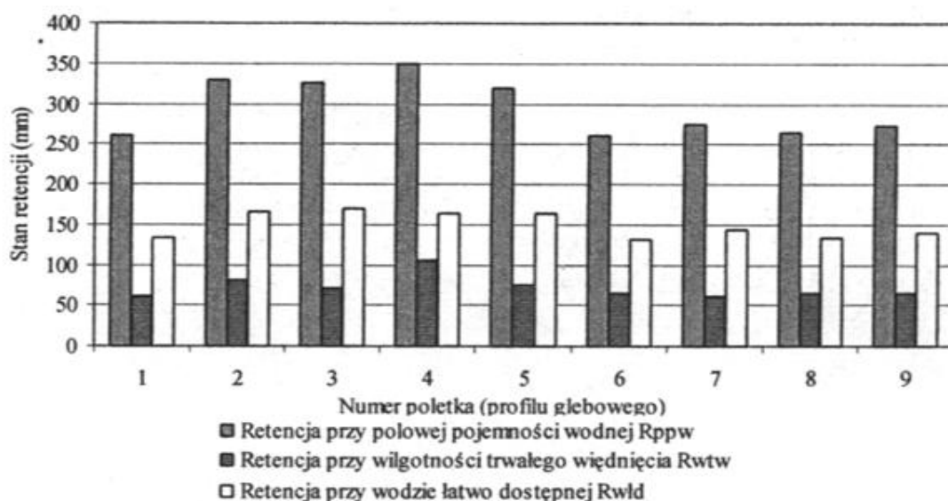
Rys 3. Wybrane właściwości wodne badanych profili gruntów pogórnich Fig. 3. Selected water properties of investigated soil profiles of former mining areas
