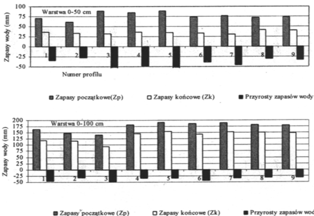
Rys. 5. Zapasy wody w mm przed (Zp) i po (Zk) okresie o niskiej sumie opadów oraz przyrosty zapasów wody w profilach gruntów pogórnicznych w roku 2001 Fig. 5. Water contents (mm) before (Zp) and after (Zk) period of low precipitation sums and increases of water contents in post-mining grounds profiles in the year 2001
