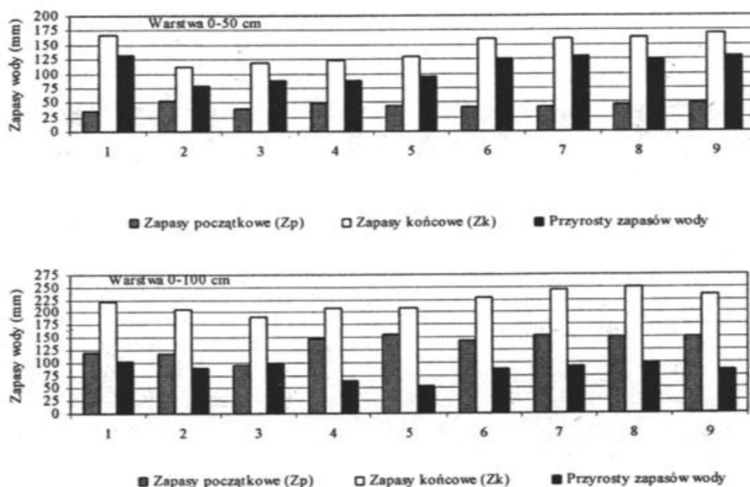
Rys. 6. Zapasy wody w mm przed (Zp) i po (Zk) okresie o wysokiej sumie opadów oraz przyrosty zapasów wody w profilach gruntów pogórnich w roku 2001
