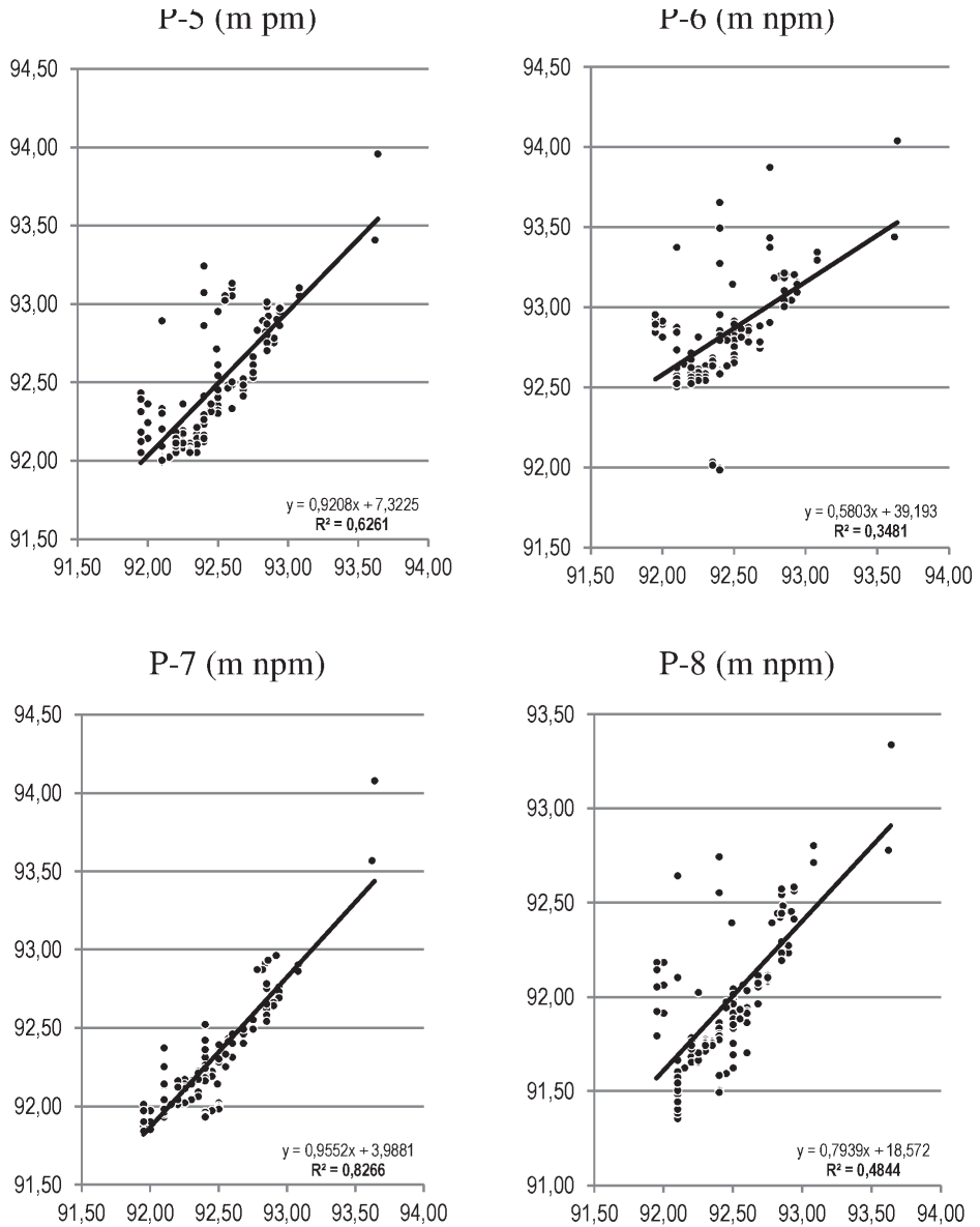
Rys. 10. Związek stanów wód w zbiorniku Pakosław ze stanami wody gruntowej w studzienkach: P-5, P-6, P-7 i P-8
