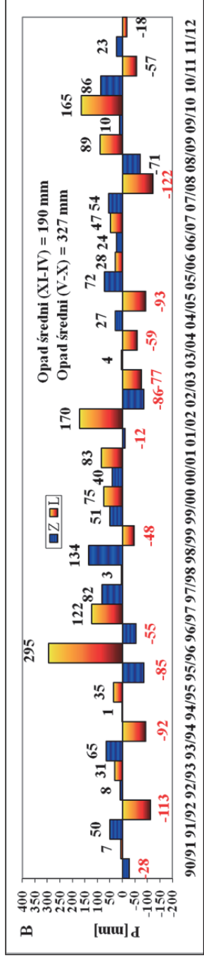
Rys. 6. Odchylenia sum opadów atmosferycznych (P) rocznych (A) i półrocznych (B) od średnich z wielolecia 1965/66–2006/2007 w analizowanych latach hydrologicznych, mierzone w posterunku opadowym KWB "Konin" w Kleczewie
